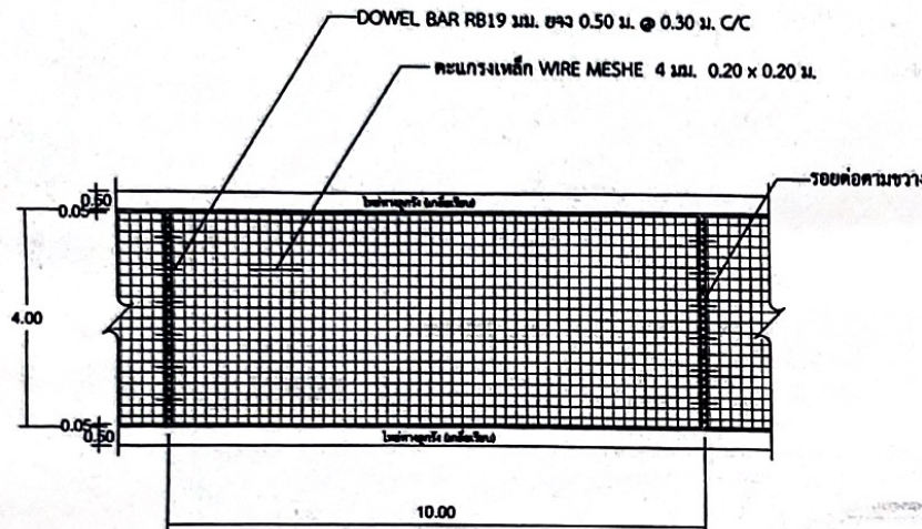
แปลนผิวจราจรคอนกรีตเสริมเหล็ก NOT TO SCALE
