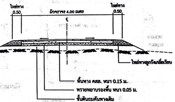
รูปตัดถนนจราจรคอนกรีตเสริมเหล็ก NOT TO SCALE
