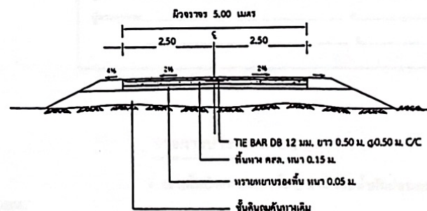
รูปตัดถนนจราจรคอนกรีตเสริมเหล็ก คสล. NOT TO SCALE
