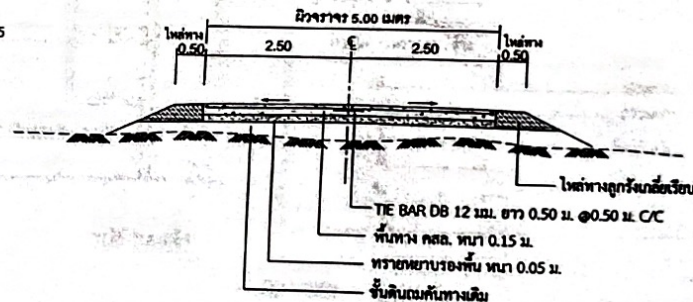
รูปตัดถนนจราจรคอนกรีตเสริมเหล็ก NOT TO SCALE
