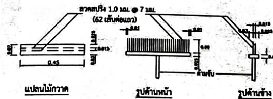
แบบขยายไม้กวาดลากผิวพื้น คสท.
